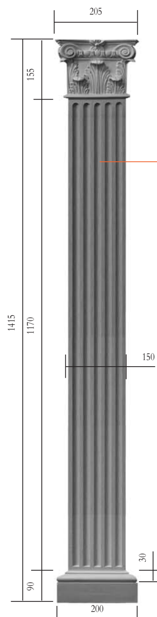
PIP 856 Pilastre à cannelures complet avec base et chapiteau 1415 x 150 x 25 mm
