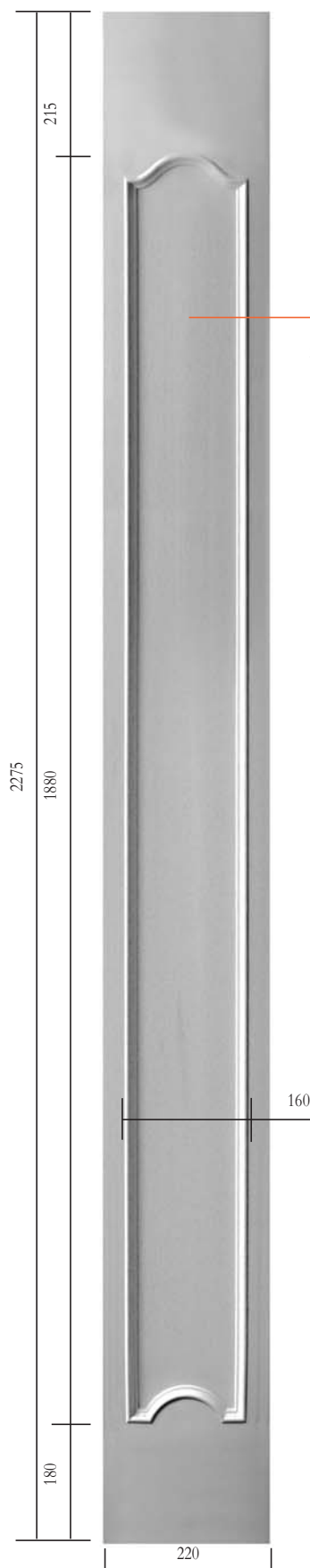
PIP 854 Pilastre complet panneau 2105 x 210 x 20 mm
