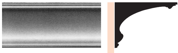
MOP 18 dimensions mur/plafond : 140 x 190 mm — longueur : 3,60 m
