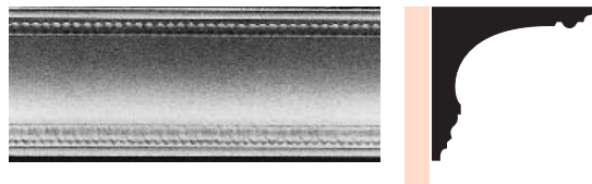
MOP 38 dimensions mur/plafond : 120 x 130 mm — longueur : 3,60 m
