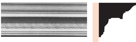
MOP 33 dimensions mur/plafond : 120 x 130 mm — longueur : 3,60 m
