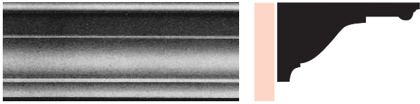
MOP 64 dimensions mur/plafond : 70 x 160 mm — longueur : 3,60 m
