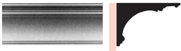
MOP 41 dimensions mur/plafond : 130 x 190 mm — longueur : 3,60 m
