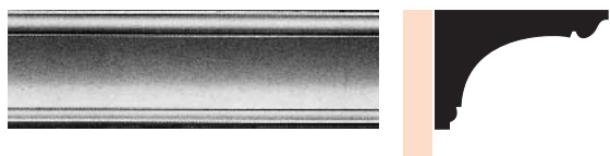
MOP 20 dimensions mur/plafond : 80 x 120 mm — longueur : 3,60 m
