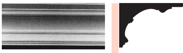
MOP 44 dimensions mur/plafond : 125 x 190 mm — longueur : 3,60 m
