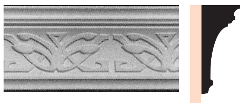
MOP 57 dimensions mur/plafond : 170 x 75 mm + 2 x 200 mm de plat — long. : 1,60
