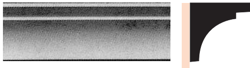
MOP 08 dimensions mur/plafond : 75 x 80 mm — longueur : 3,20 m
