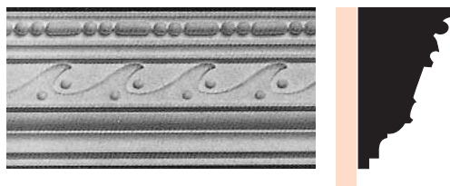
MOP 59 dimensions mur/plafond : 155 x 90 mm — longueur : 2,55 m
