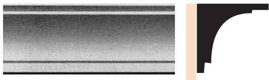
MOP 02 dimensions mur/plafond : 145 x 150 mm — longueur : 3,60 m
