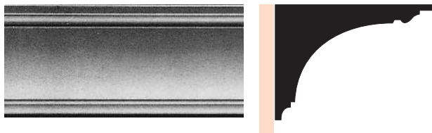
MOP 12 dimensions mur/plafond : 160 x 225 mm — longueur : 3,60 m
