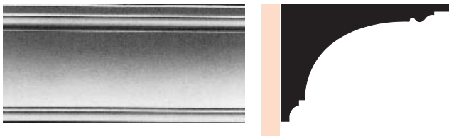
MOP 27 dimensions mur/plafond : 125 x 180 mm — longueur : 3,60 m
