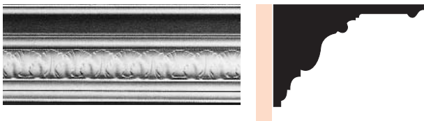
MOP 30 dimensions mur/plafond : 125 x 190 mm — longueur : 3,60 m
